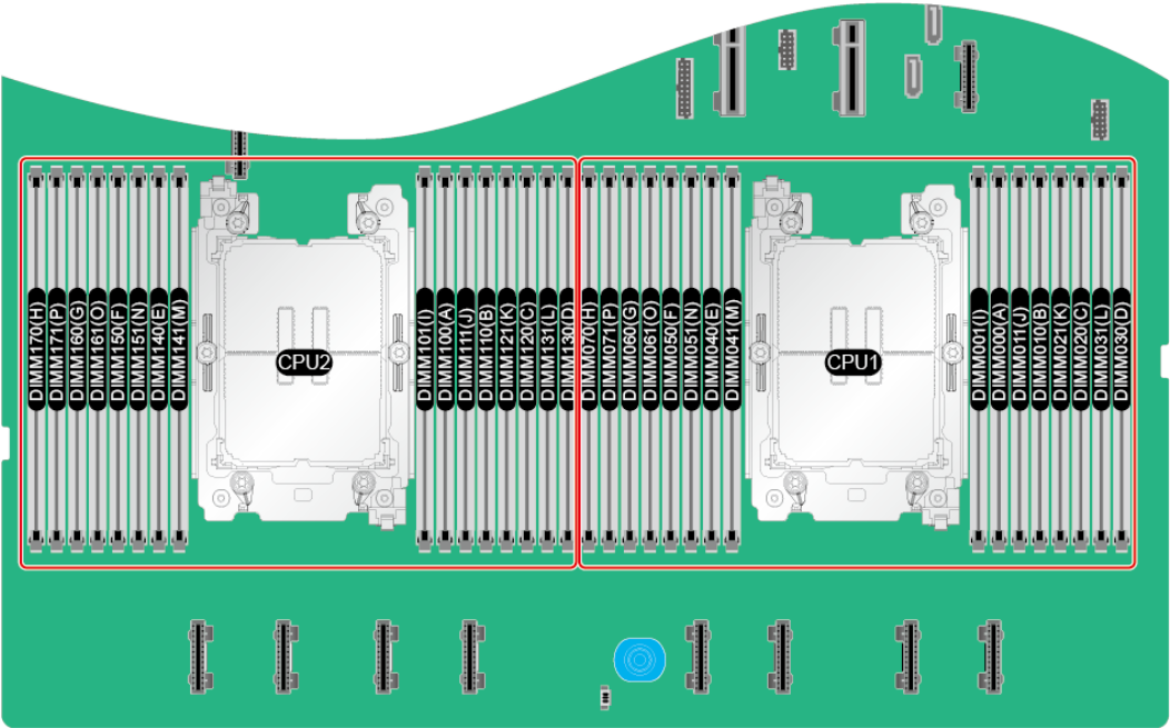
图 5-15 内存插槽位置
