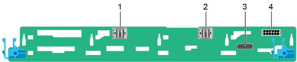
图 5-35 8x2.5 英寸硬盘直通配置背板
