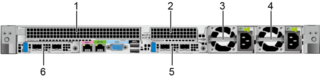
图 5-10 后面板外观
