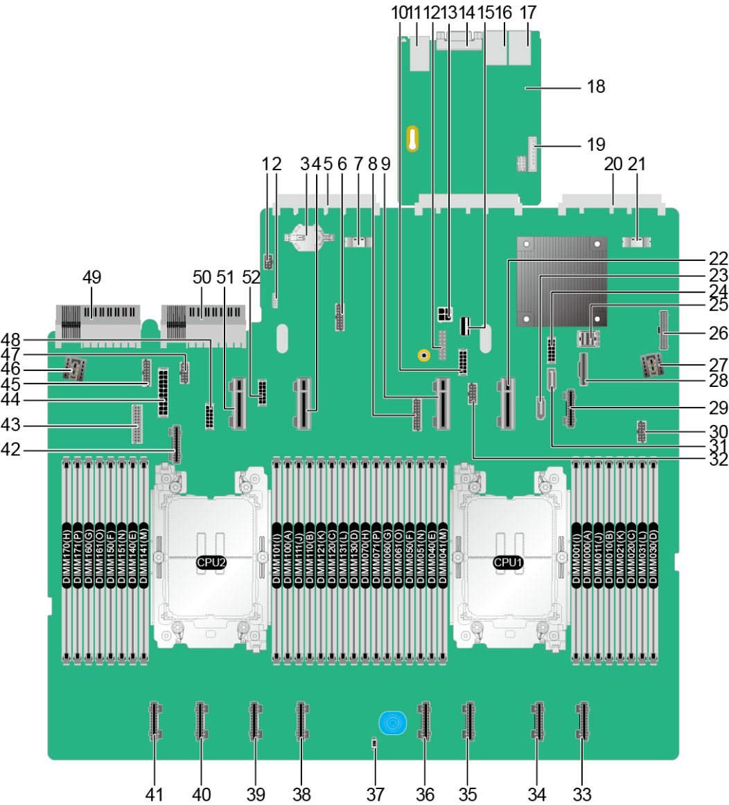
图 5-33 主板
