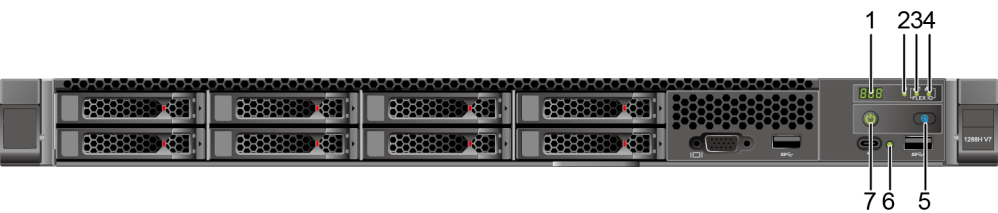
图 5-5 前面板指示灯和按钮
