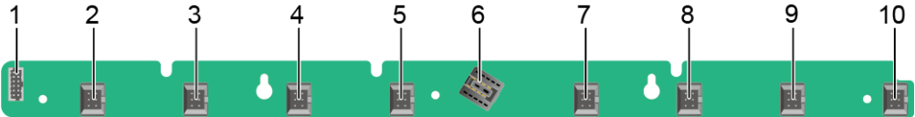
图 5-39 风扇板
