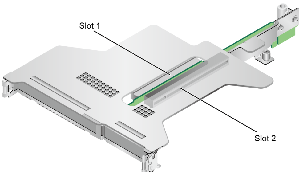
图 5-29 IO 模组 1
