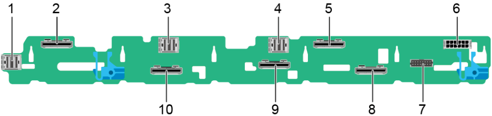
图 5-37 10x2.5 英寸硬盘 NVMe 配置背板
