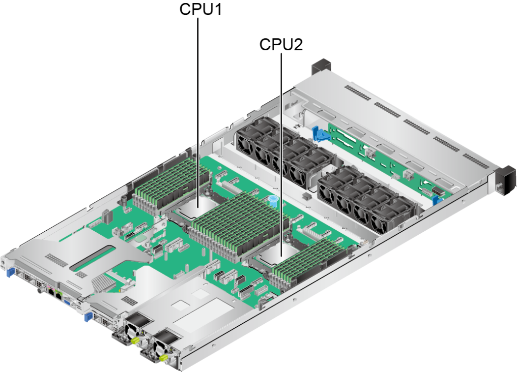
图 5-13 处理器位置
