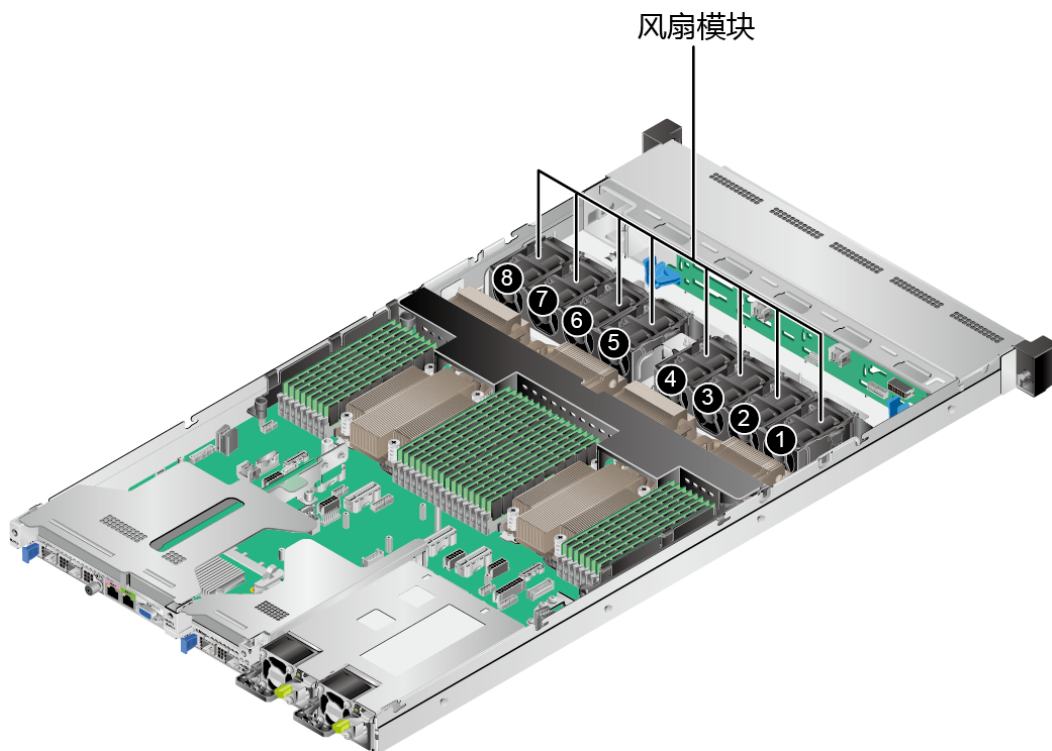
图 5-32 风扇模块的位置
