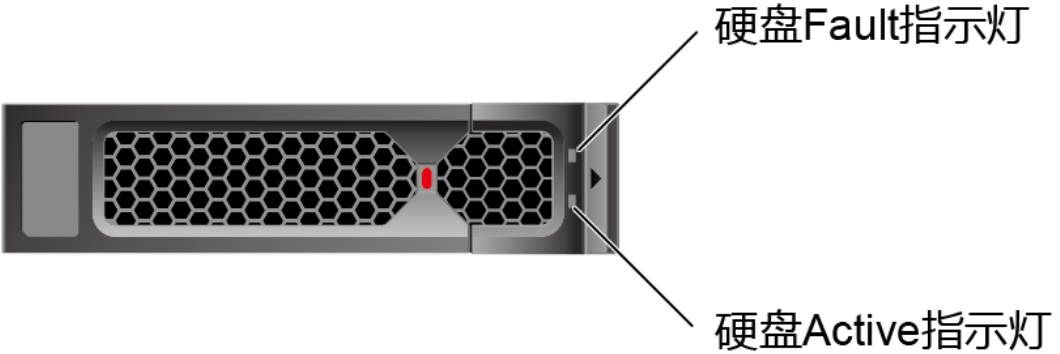
图 5-26 SAS/SATA 硬盘指示灯
