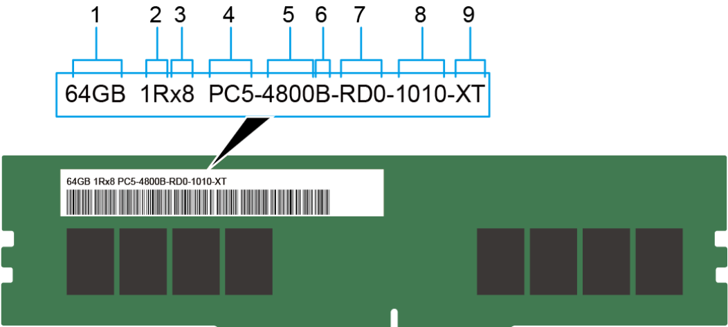
图 5-14 内存标识
