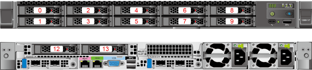
图 5-24 硬盘编号
