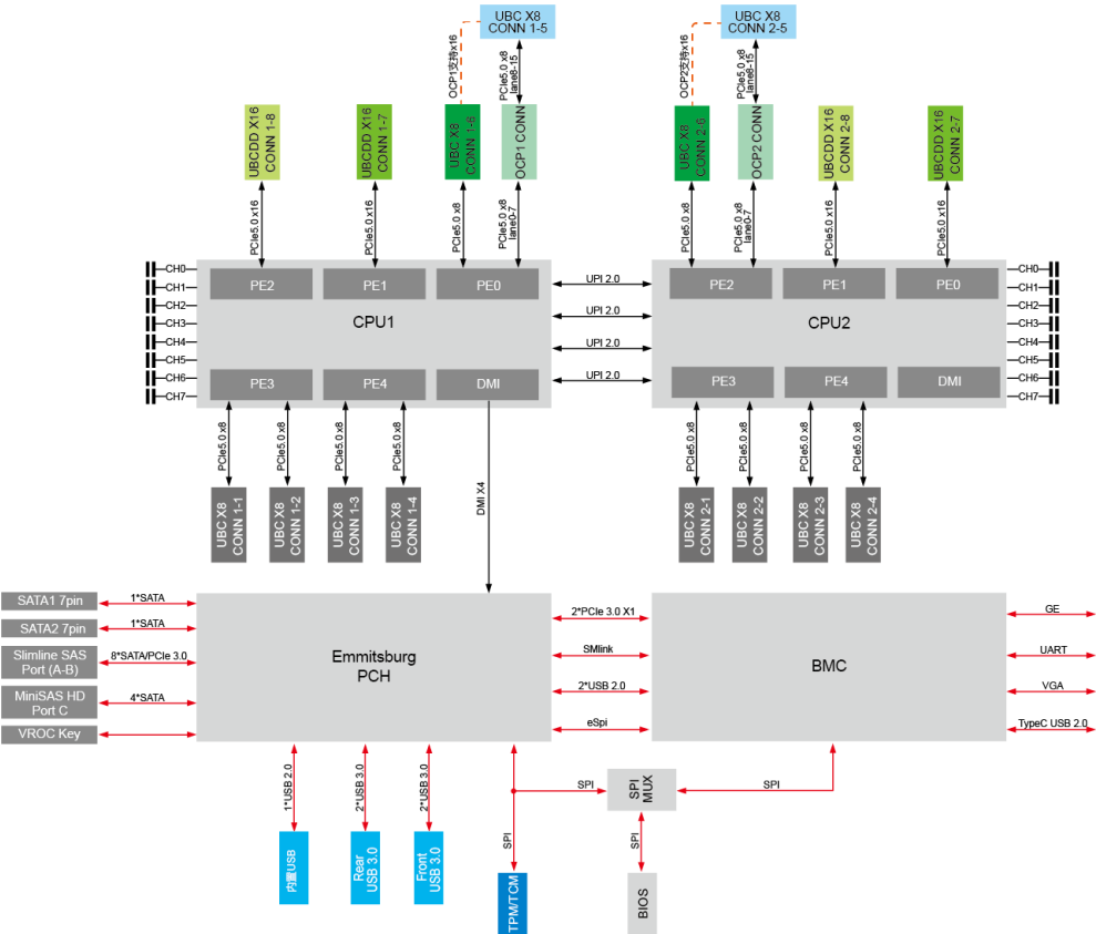
图 4-1 逻辑结构
