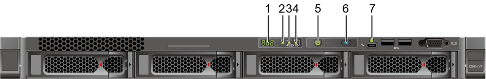
图 5-4 前面板指示灯和按钮
