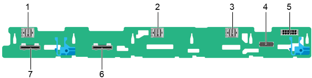
图 5-36 10x2.5 英寸硬盘直通配置背板
