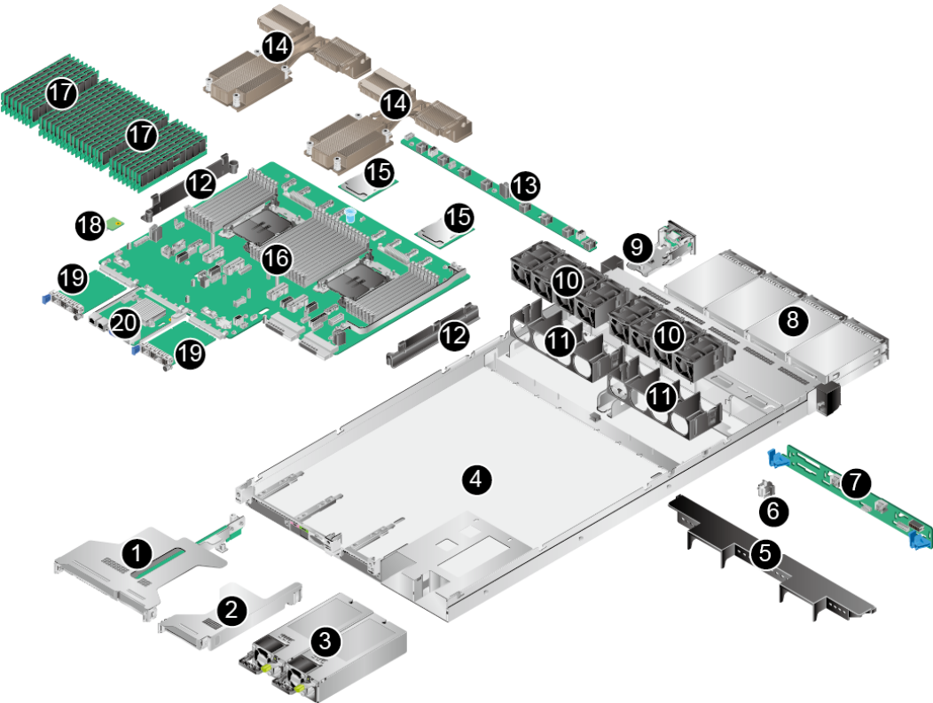
图 3-1 物理结构（示例：8x2.5 英寸硬盘配置）
