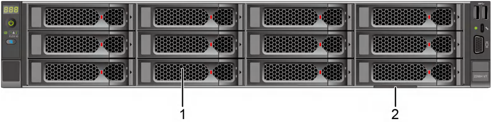
图 5-3 前面板外观
