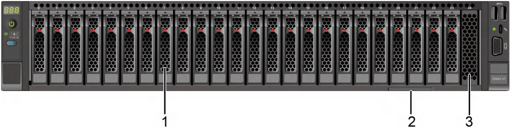
图 5-4 前面板外观
