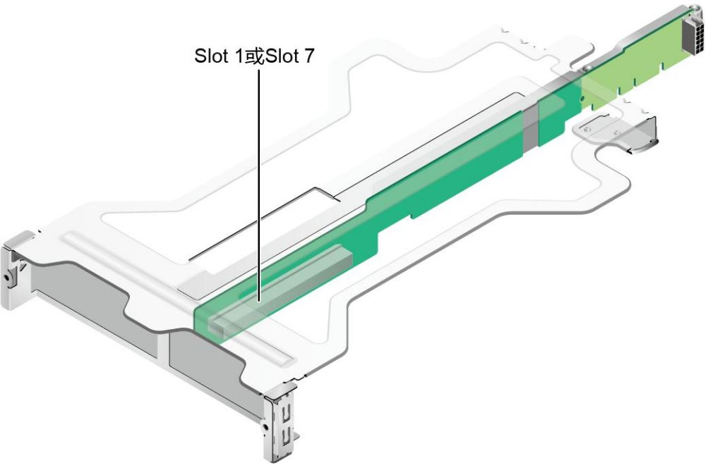
图 5-63 PCIe Riser 卡 3
