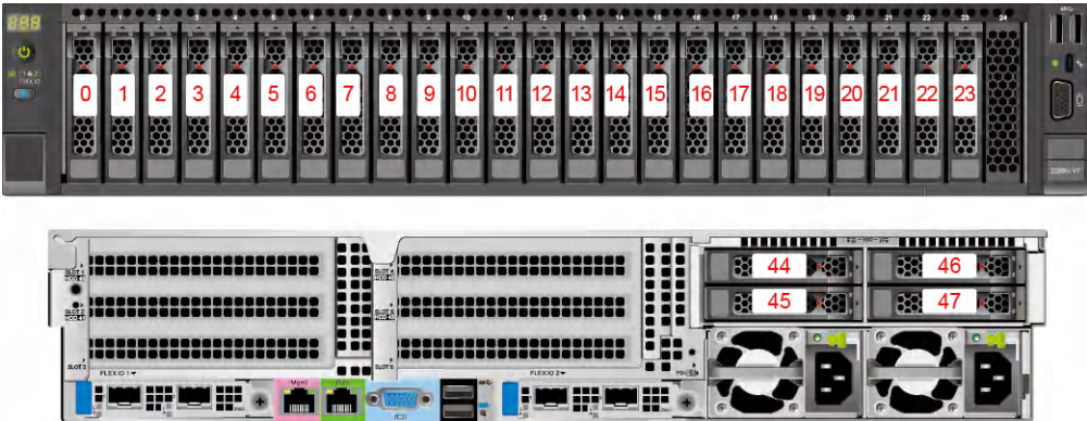
图 5-46 硬盘编号
