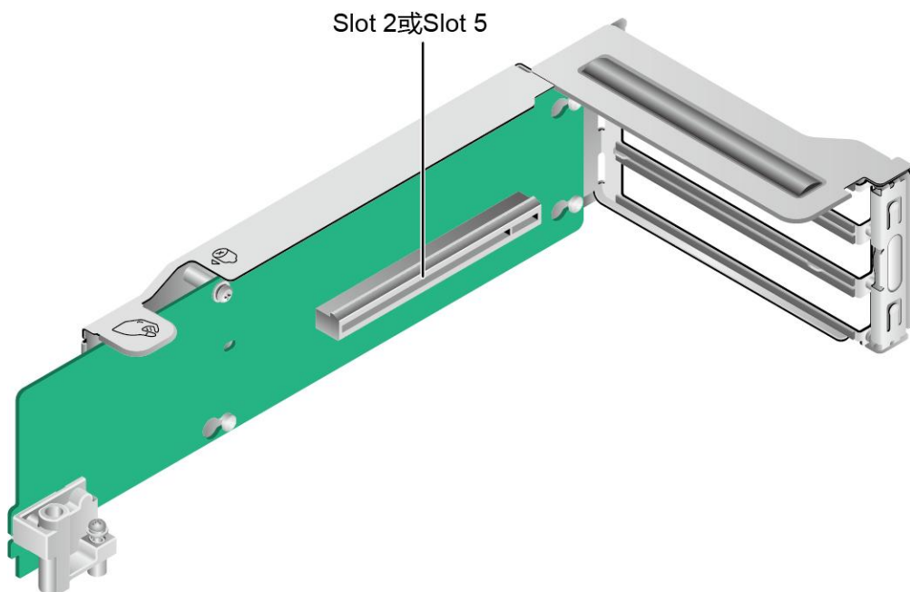
图 5-58 PCIe Riser 卡 5
