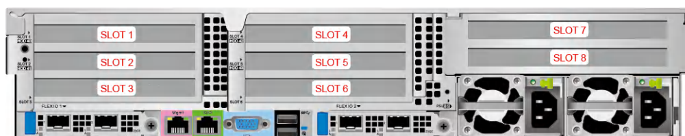
图 5-51 PCIe 插槽
