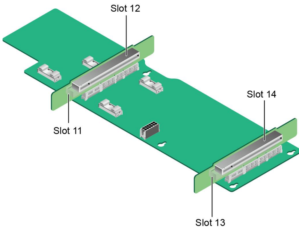
图 5-61 PCIe Riser 卡 1
