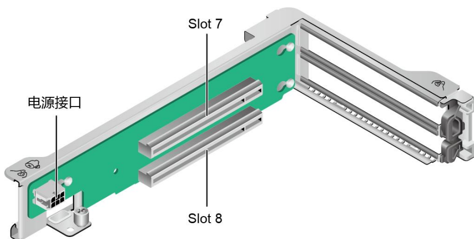
图 5-59 PCIe Riser 卡 1
