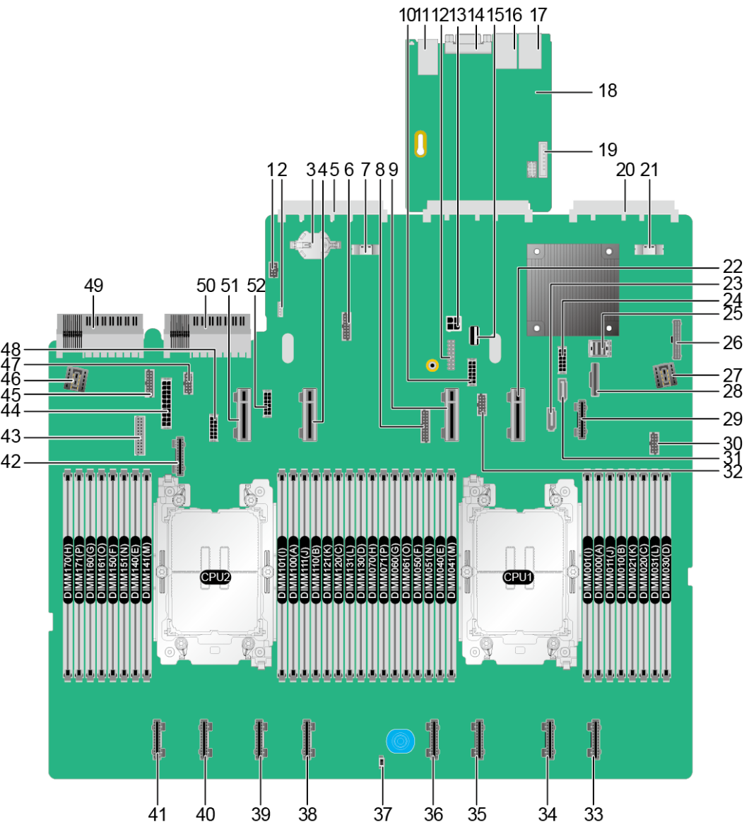
图 5-68 主板
