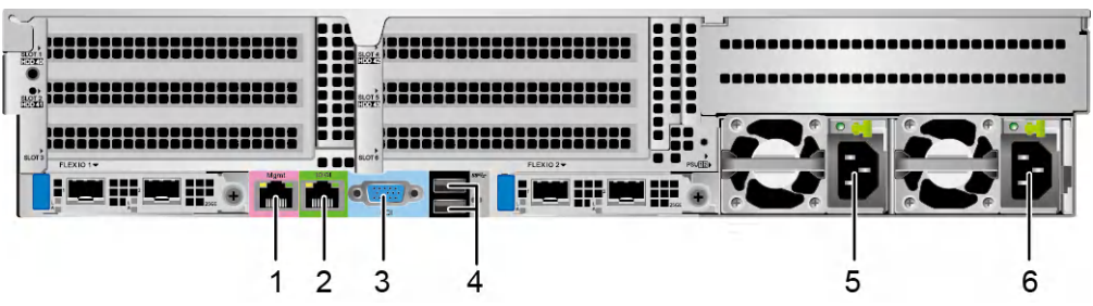
图 5-20 后面板接口
