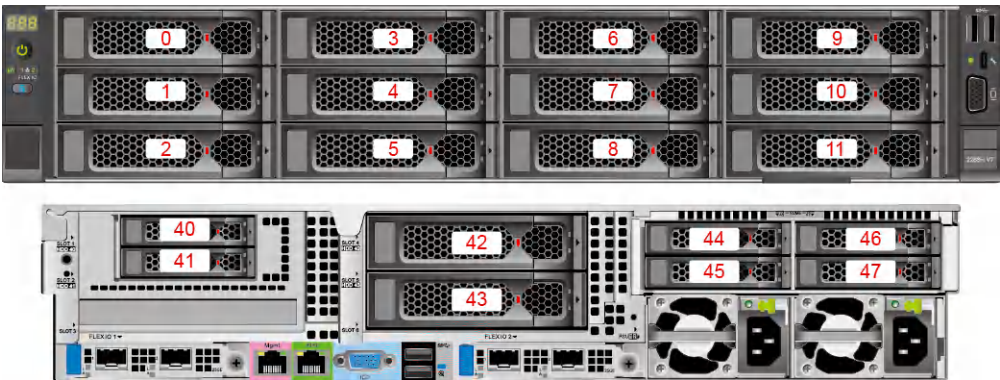
图 5-41 硬盘编号
