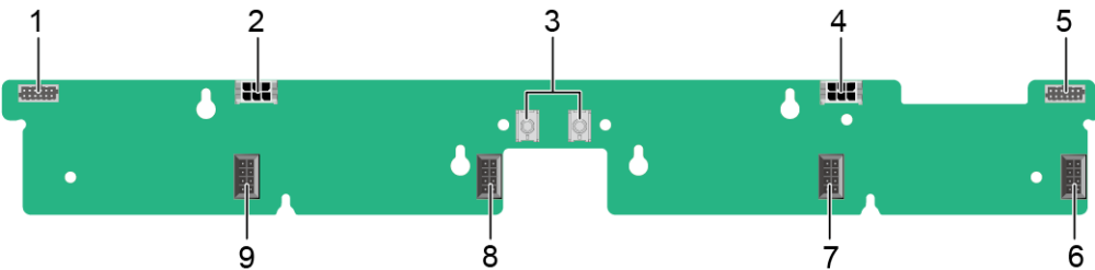
图 5-81 风扇板
