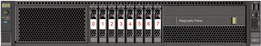
图 5-33 硬盘编号
