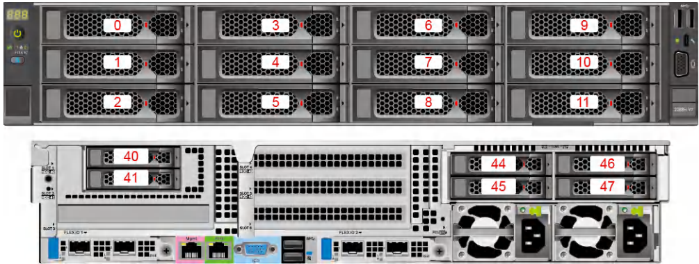
图 5-37 硬盘编号（IO 模组 1 配置 2.5 英寸硬盘）
