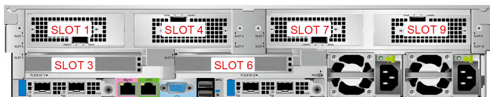
图 5-52 PCIe 插槽
