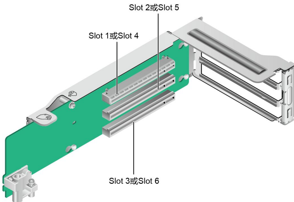
图 5-54 PCIe Riser 卡 1
