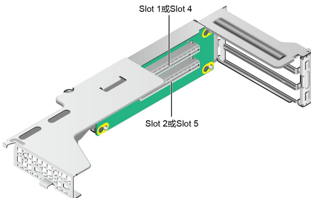
图 5-55 PCIe Riser 卡 2
