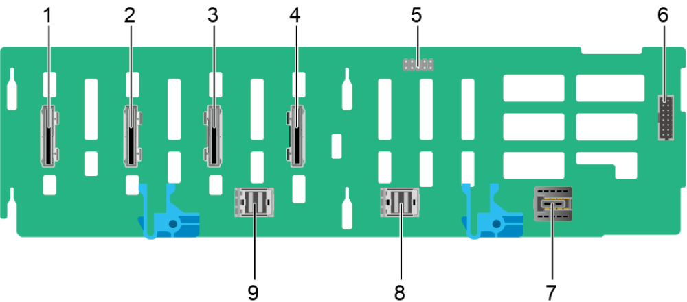
图 5-71 12x2.5 英寸硬盘直通配置（4xSAS/SATA+8xNVMe）背板
