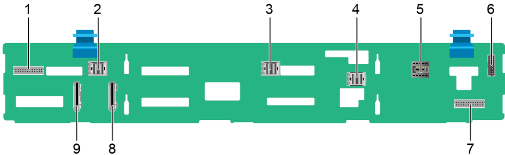
图 5-72 12x3.5 英寸硬盘直通配置背板
