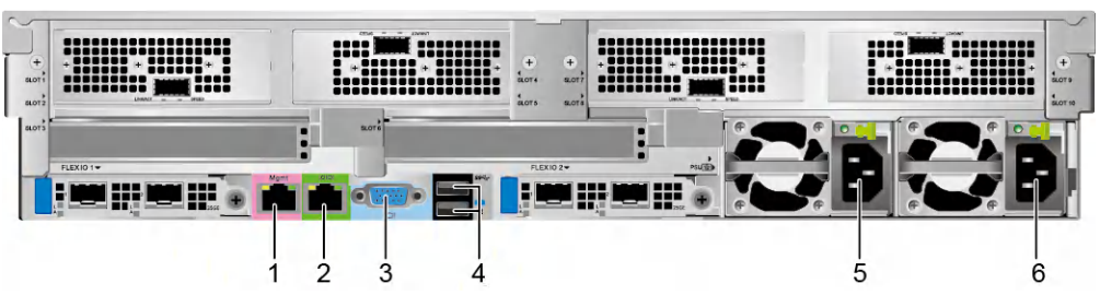
图 5-21 后面板接口
