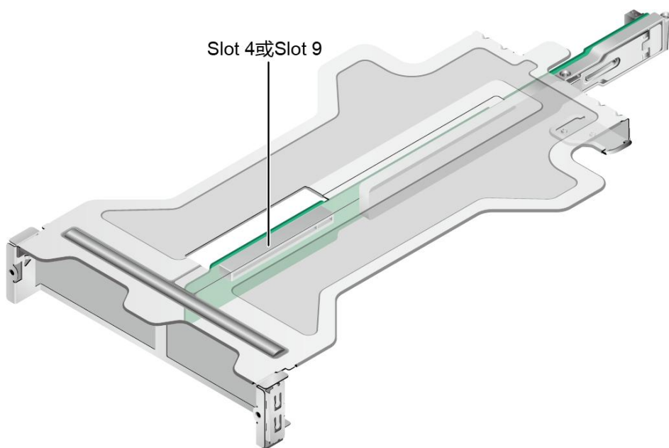
图 5-62 PCIe Riser 卡 2
