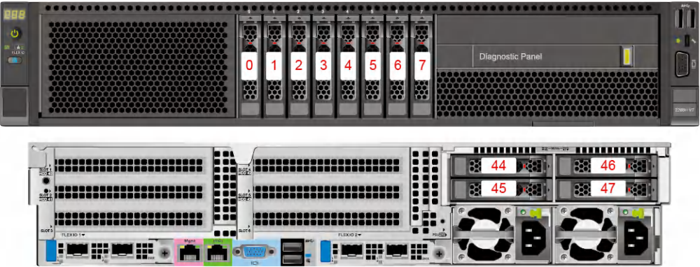
图 5-29 硬盘编号
