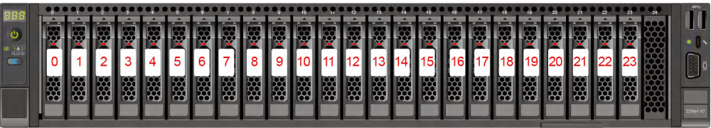
图 5-44 硬盘编号
