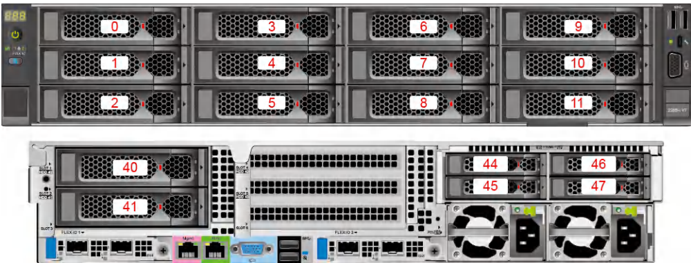
图 5-40 硬盘编号
