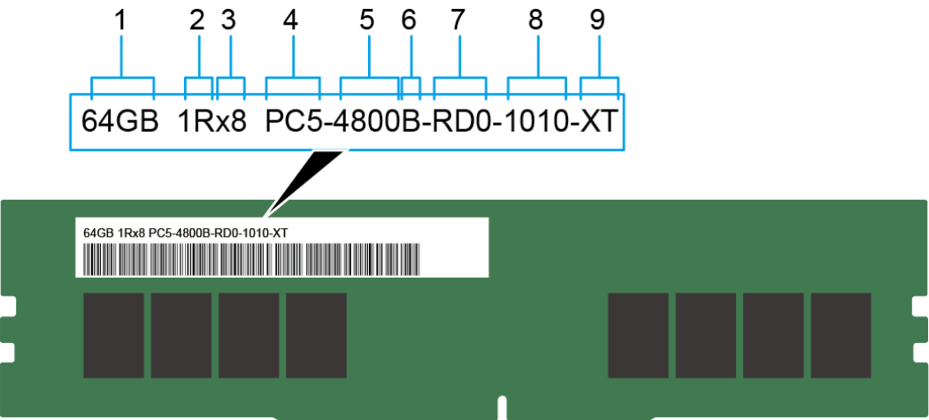
图 5-23 内存标识
