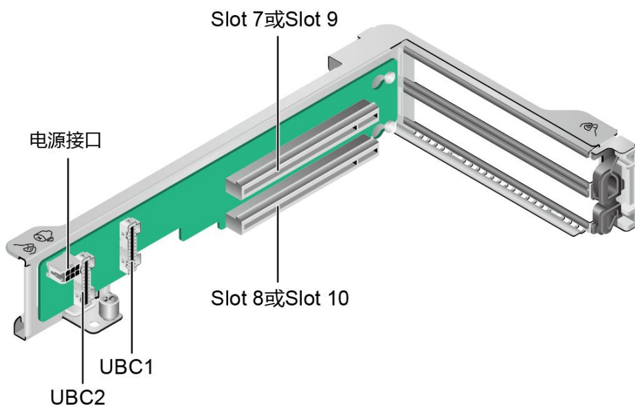
图 5-60 PCIe Riser 卡 2
