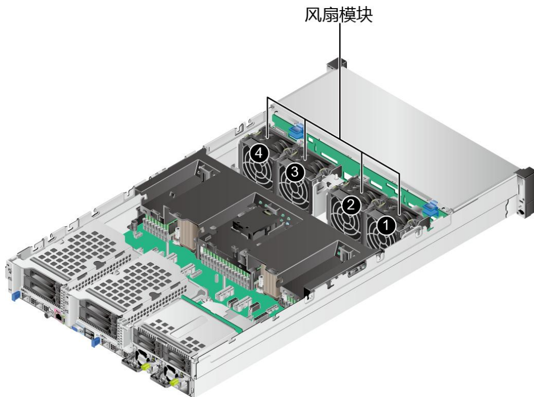
图 5-65 风扇模块的位置
