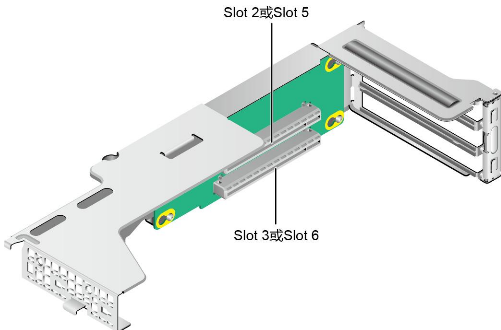
图 5-56 PCIe Riser 卡 3
