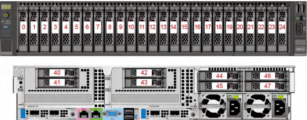
图 5-48 硬盘编号
