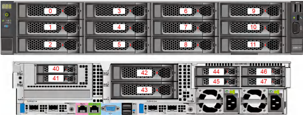
图 5-39 硬盘编号
