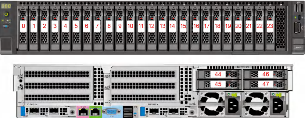
图 5-43 硬盘编号
