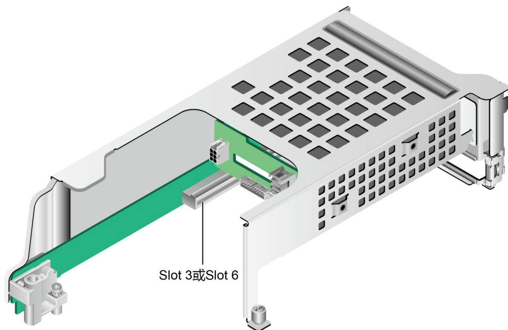
图 5-57 PCIe Riser 卡 4
