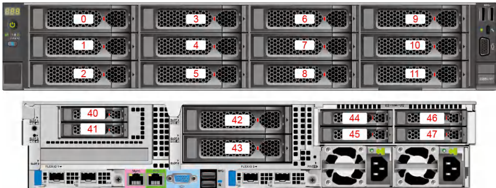
图 5-42 硬盘编号
