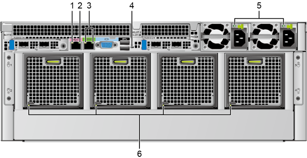
图 5-5 后面板指示灯
