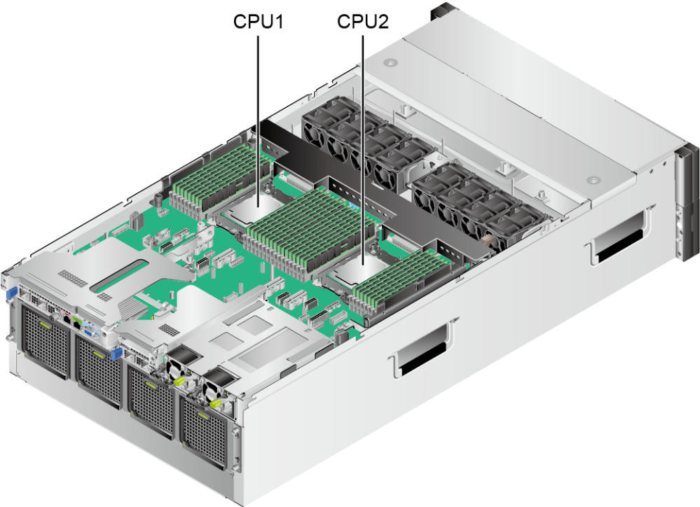
图 5-7 处理器位置
