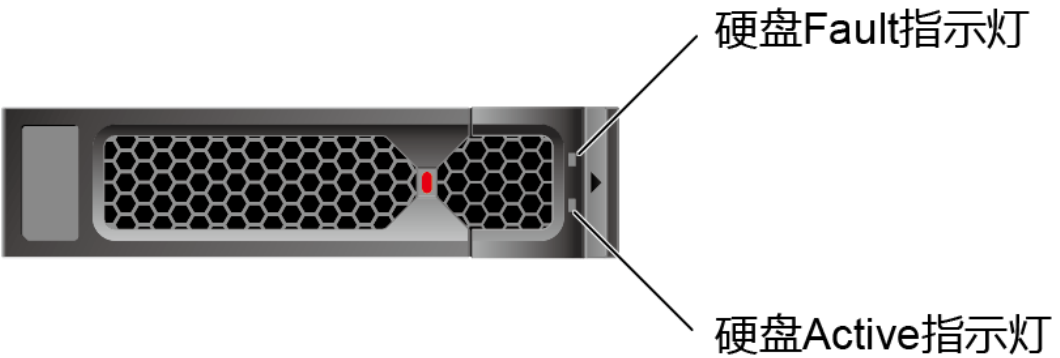
图 5-20 NVMe 硬盘指示灯
