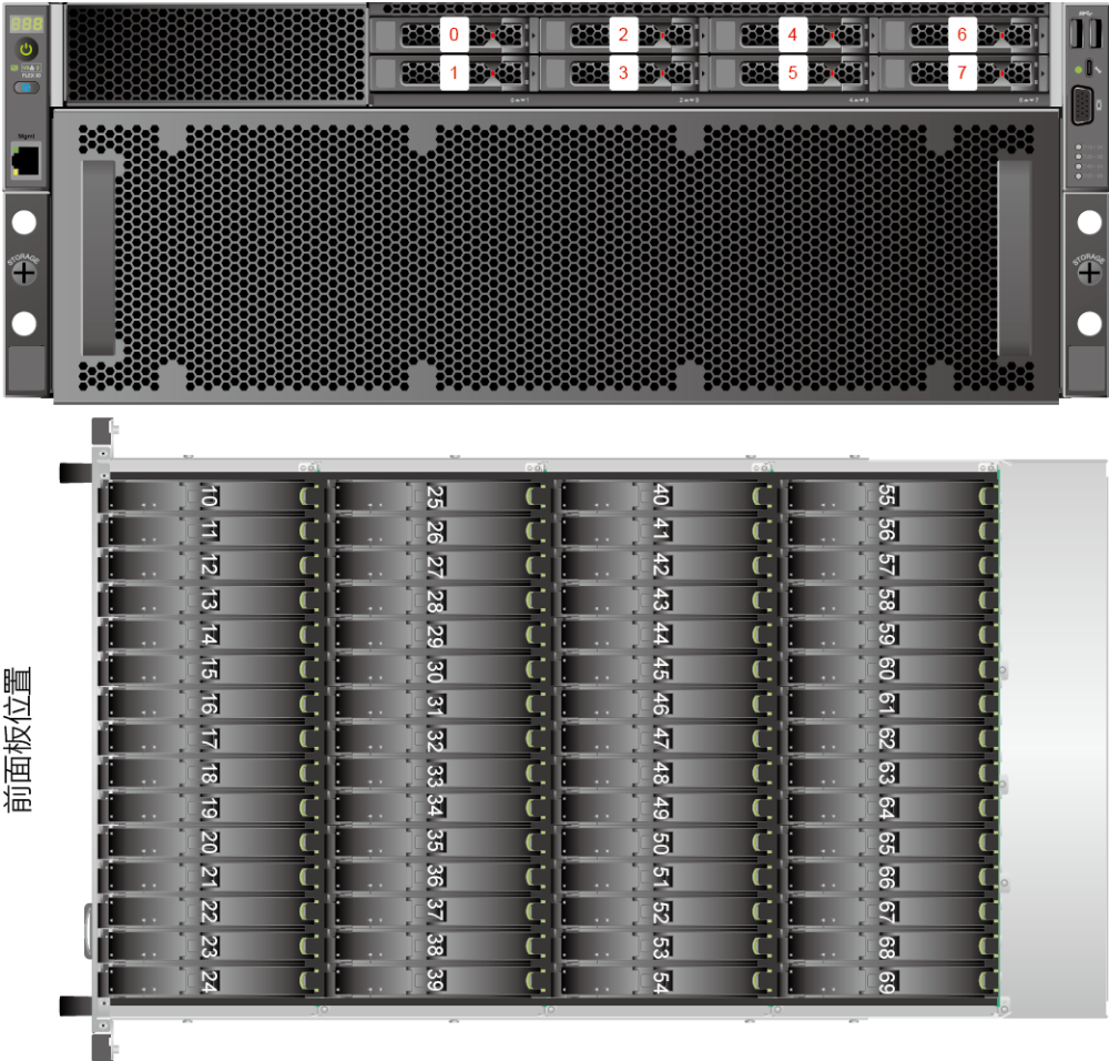
图 5-15 硬盘编号
