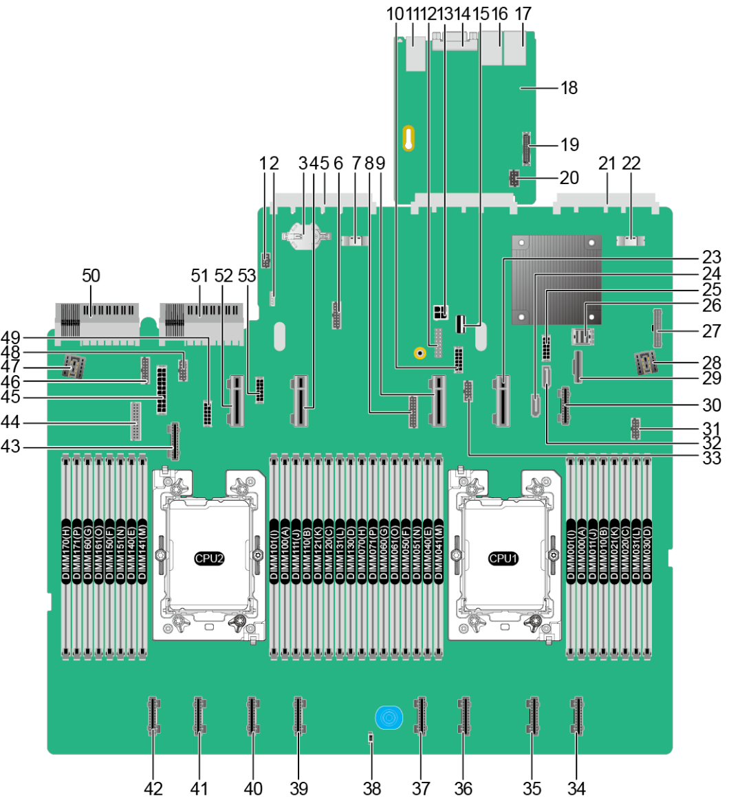
图 5-27 主板
