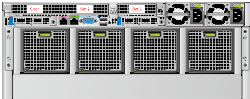
图 5-21 PCIe 插槽
