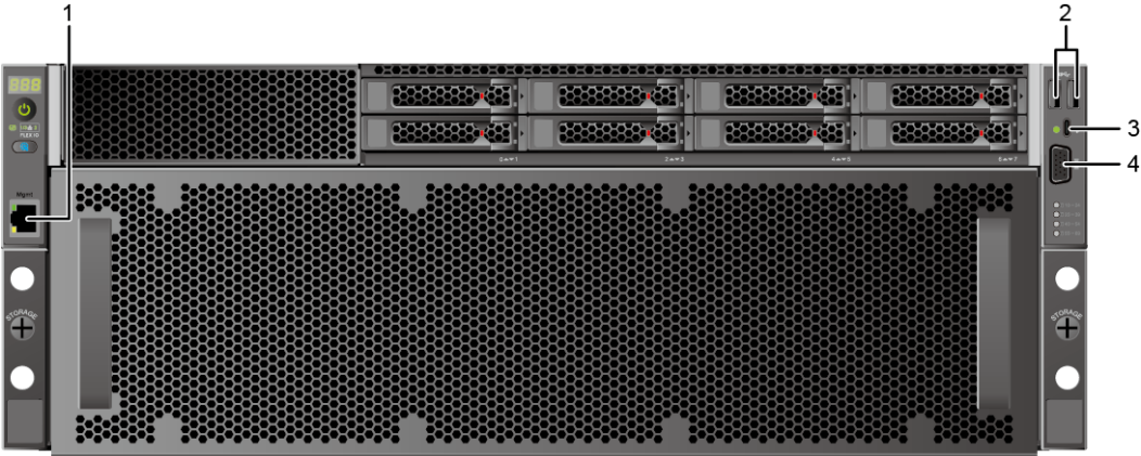
图 5-3 前面板接口
