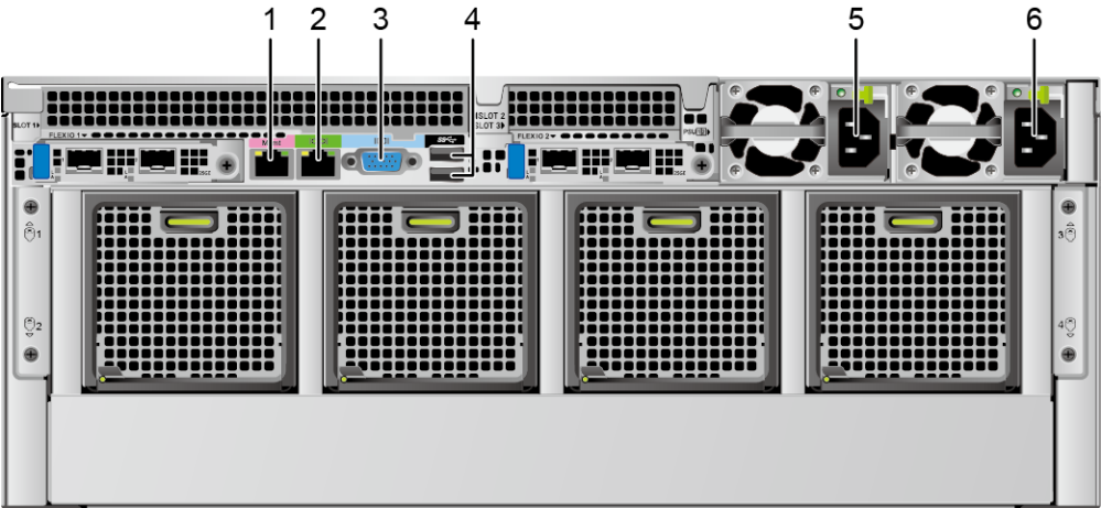
图 5-6 后面板接口
