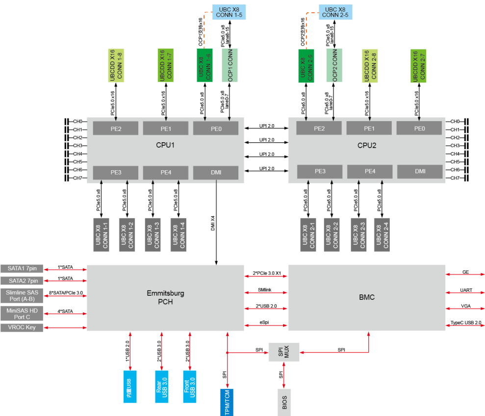
图 4-1 逻辑结构
