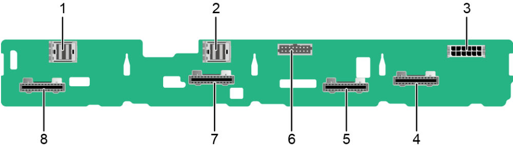
图 5-28 8x2.5 英寸硬盘背板
