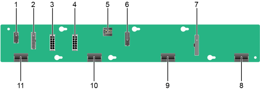
图 5-31 后置风扇板
