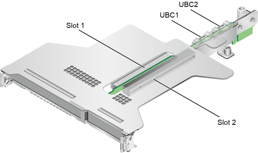
图 5-22 IO 模组 1
