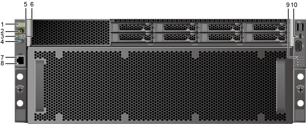
图 5-2 前面板指示灯和按钮
