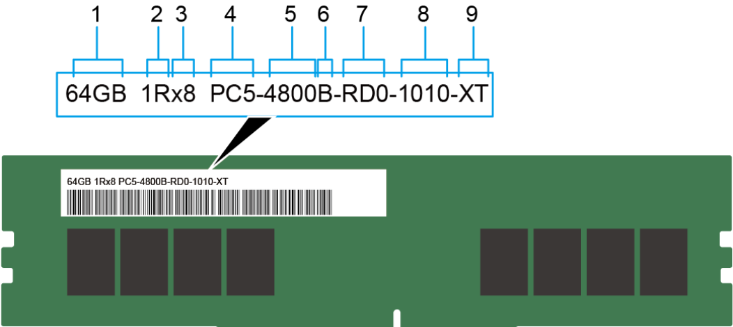
图 5-8 内存标识
