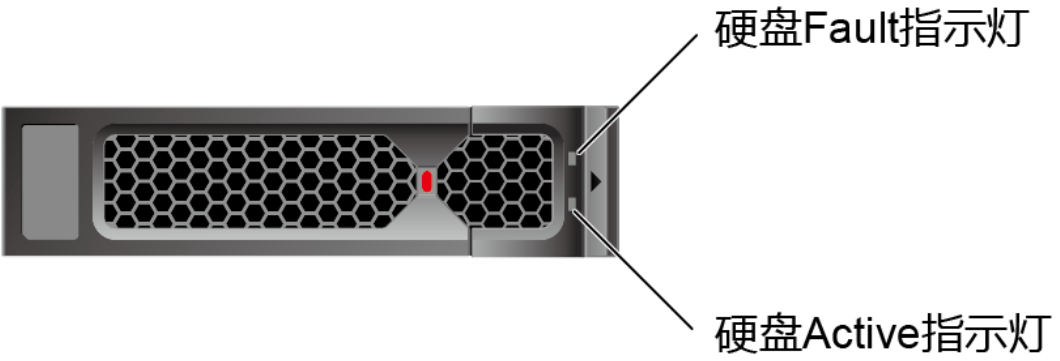
图 5-18 SAS/SATA 硬盘指示灯（前置硬盘）
