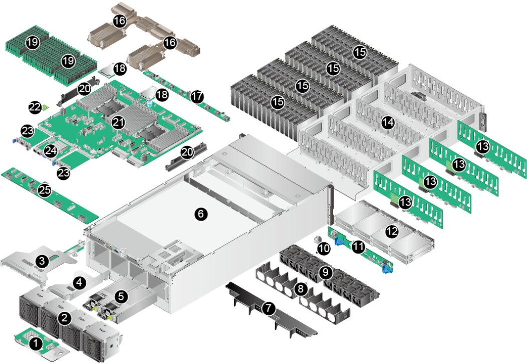
图 3-1 物理结构
