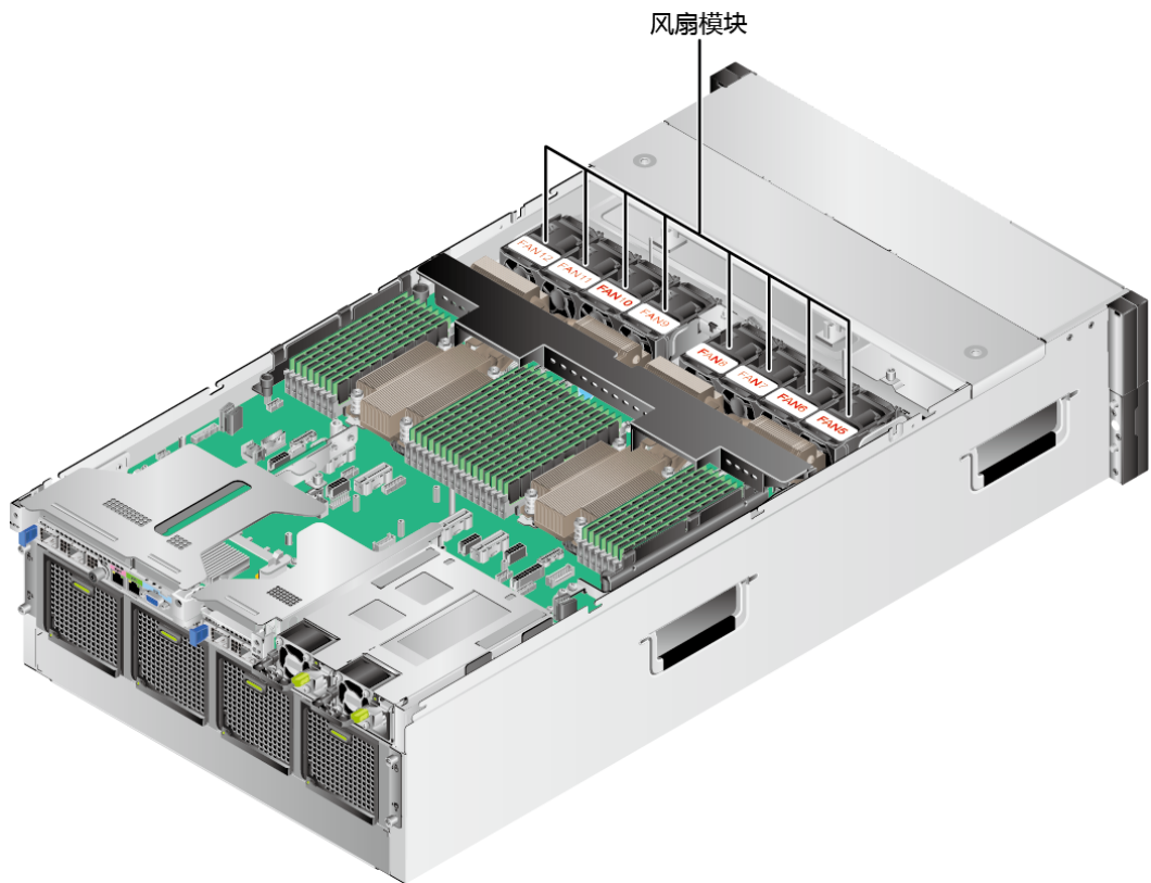
图 5-26 内置风扇模块的位置
