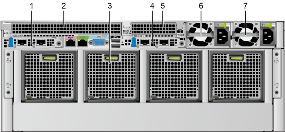
图 5-4 后面板外观
