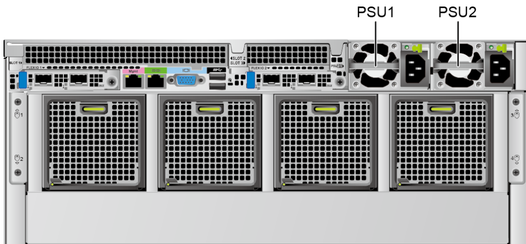
图 5-24 电源模块位置
