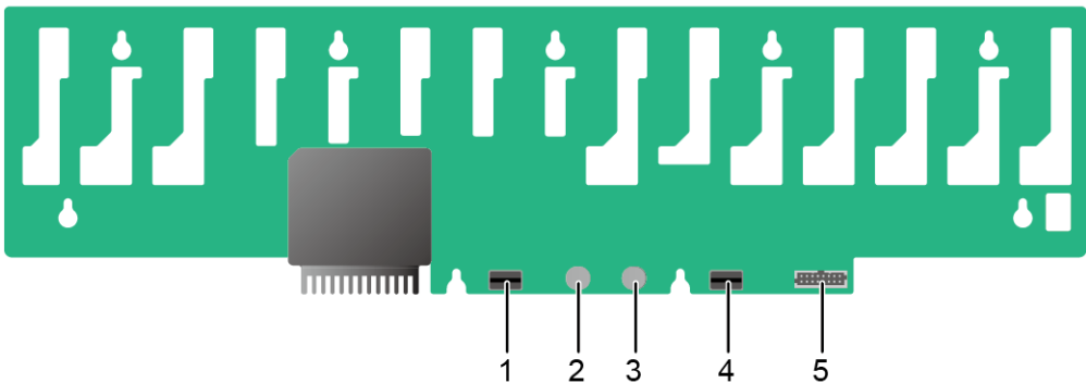
图 5-29 15x3.5 英寸硬盘背板
